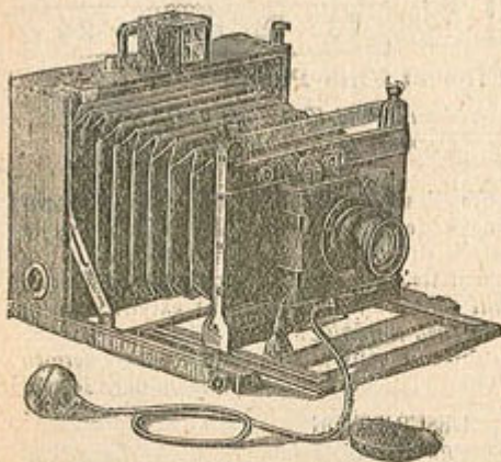
Fig. 100. — Appareil ouvert
